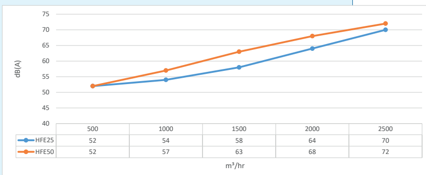
* grafiek geluidsniveau HFE-25 en HFE-50
